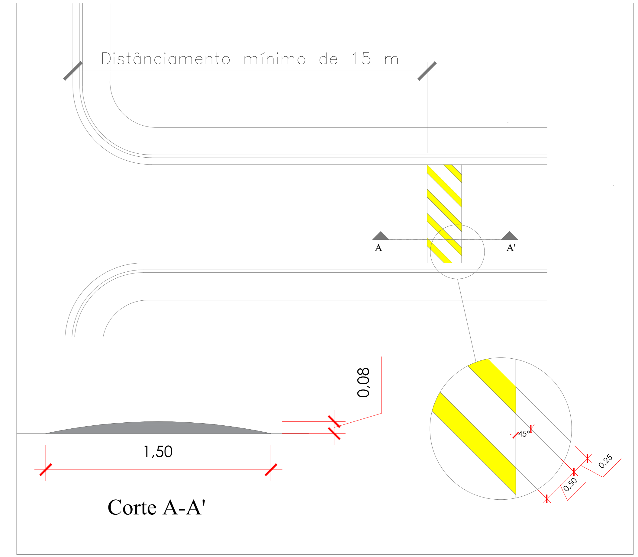
DETALHE LOMBADA S / ESCALA
