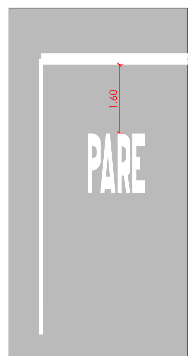
LRE - Linha de Retenção (esp.:0,30m)
