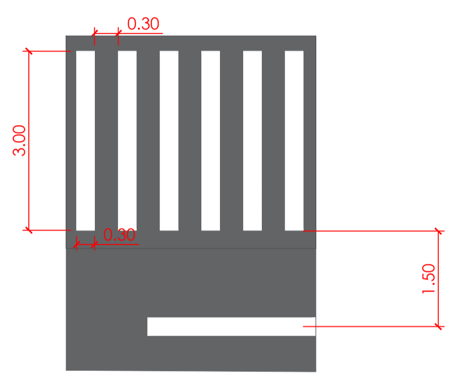
Detalhe Pintura de Sinalização Horizontal
